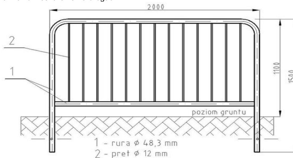
Ogrodzenie segmentowe U-12a (rurowe).
